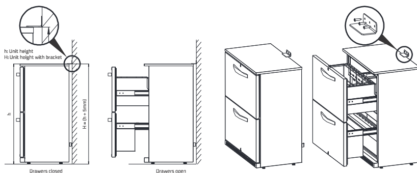
BEVESTIGINGSBEUGEL PLAATSEN OPTIE 2
