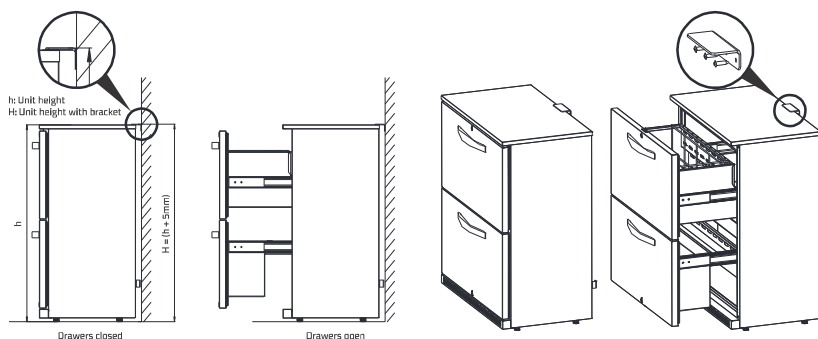
BEVESTIGINGSBEUGEL PLAATSEN OPTIE 1
